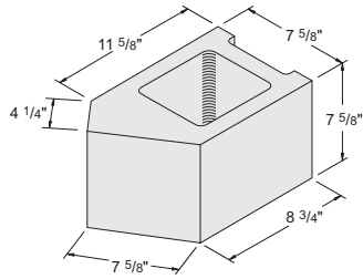
8" 45° Angle #1030130
