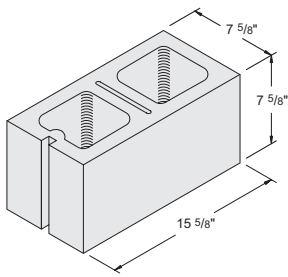
8" x 8" x 16" Splitable Jamb #1030010
