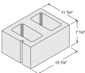
12" x 8" x 16" Jamb #1010020
