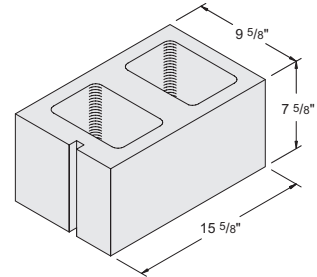
10" x 8" x 16" Jamb #1020030
