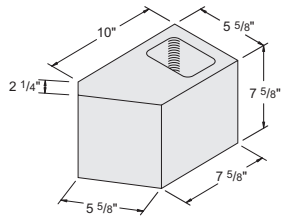
6" 45° Angle #1040280
