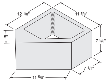
12" 45° Angle #1010140
