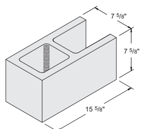
8" x 8" x 16" Conduit Item #1030300 108 units / pallet • 33 lbs. / unit
