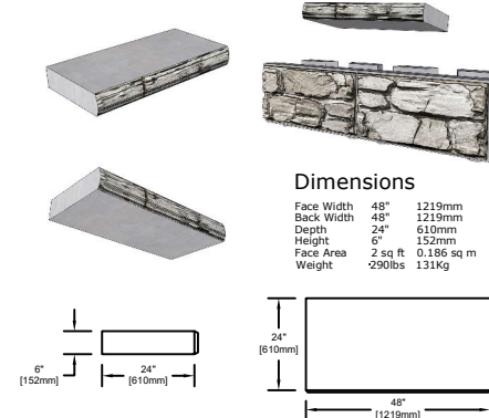
CAP UNIT
